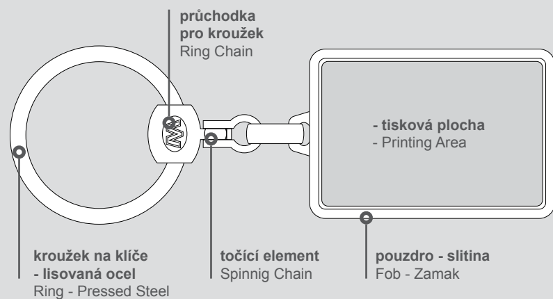
3D etiketa na jedné straně domed label on one side
