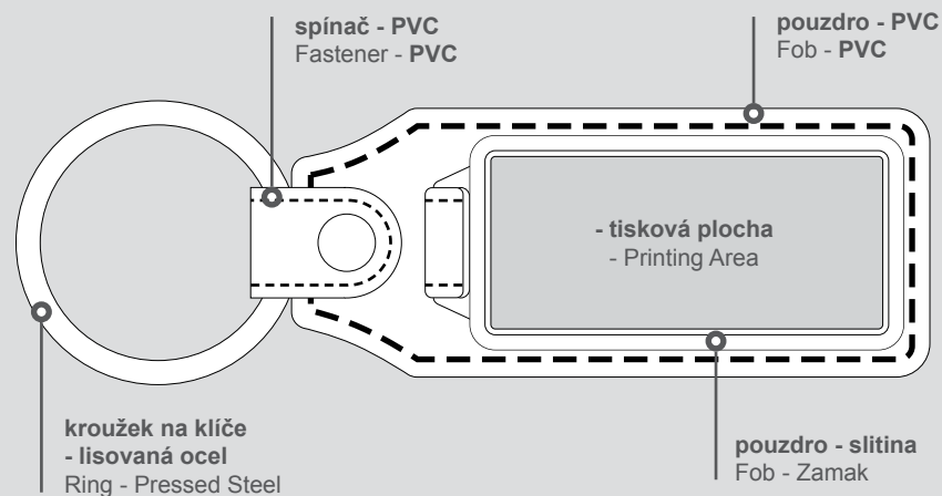
3D etiketa na jedné straně domed label on one side
